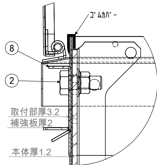
詳細図 A スケール 1 : 2
